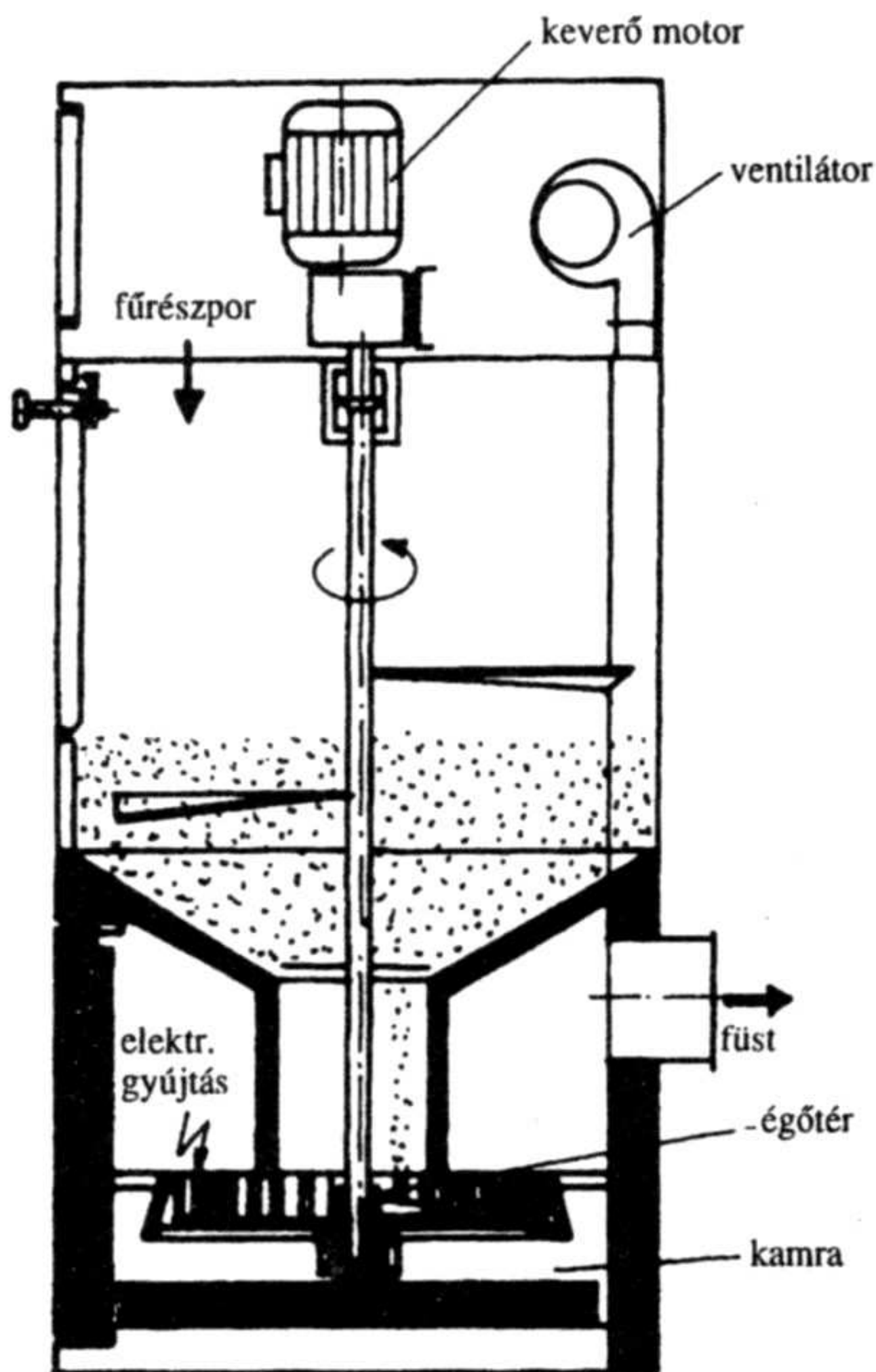
158. ábra. Izzításos fűrészporos füstgenerátor
