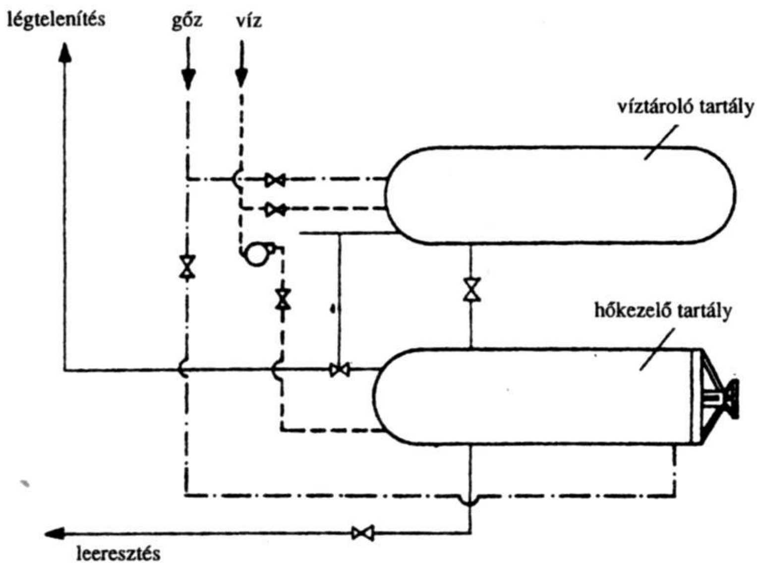
169. ábra. Fekvő autokláv
