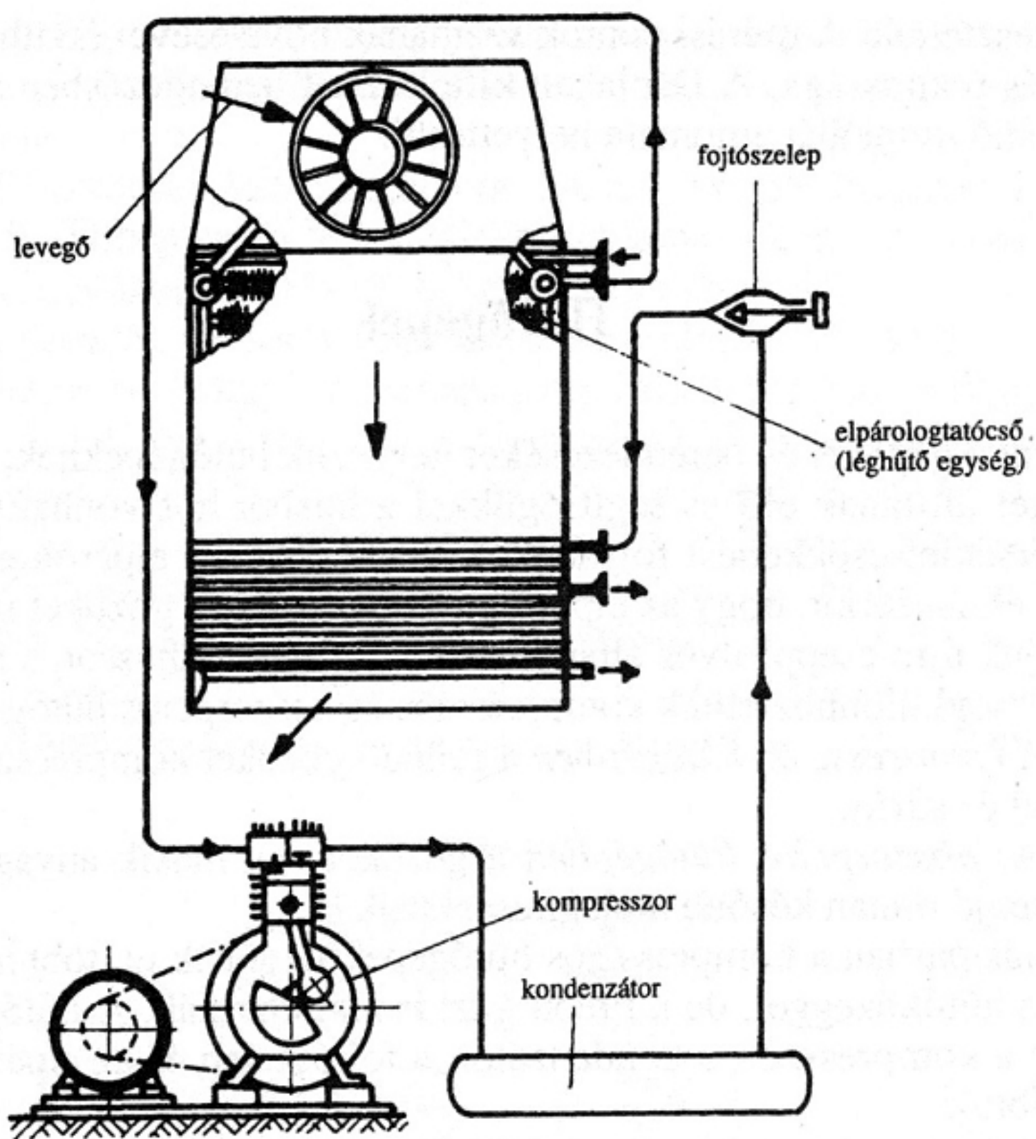
63. ábra. Hűtőkörfolyamat (nagyított léghűtő-egységgel)
