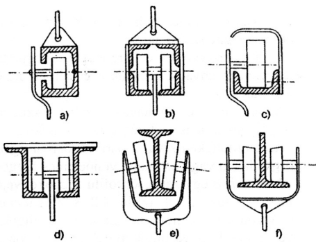
64. ábra. Magaspálya-szerkezetek a) kettős U, b) négyes L, c) U-tartó, d) kettős Z, e) I-gerenda, f) T-tartó
