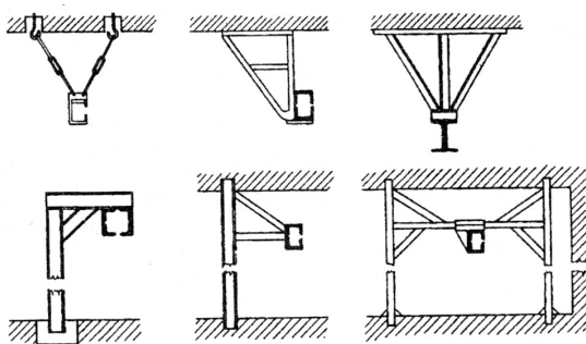
67. ábra. Baromfikonvejlör felfüggesztő szerkezetek
