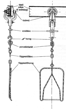
63. ábra. I-gerenda-pálya baromfi-függesztővel
