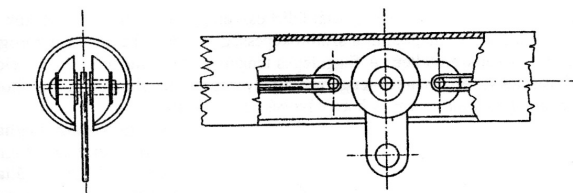
65. ábra. Csőben vezetett konvejlánc
