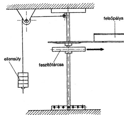
68. ábra. Ellensúlyos feszítőmű
