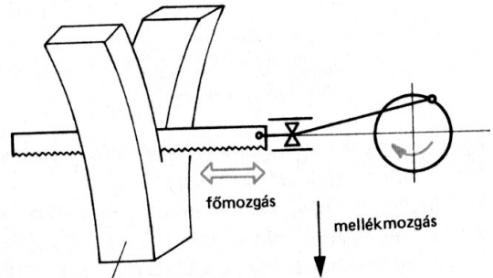
59. ábra. Váltakozó mozgású fűrész
