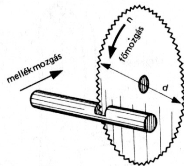
61. ábra. Körmozgású fűrész
